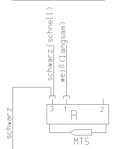
Anschlußbild Vorwiderstand
